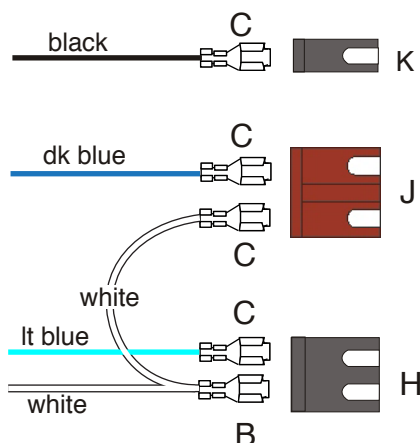
64-65 Chevelle 2 spd. connection
