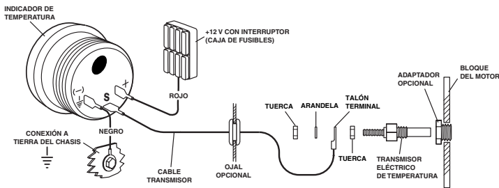
Figura 6. Conexiones del indicador eléctrico de temperatura de agua
