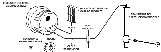
Figura 7. Conexiones del indicador eléctrico del nivel de combustible
